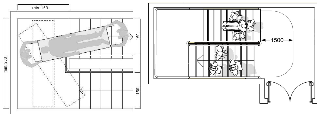
5A. ábra: Kerekesszékekkel és hordágyal történő mentésre alkalmas lépcsőház minimális méretei
