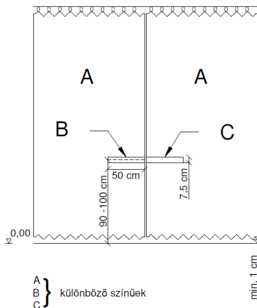
3B ábra: Fügönyök belső csatlakozó éleinek megkülönböztető jelölése
