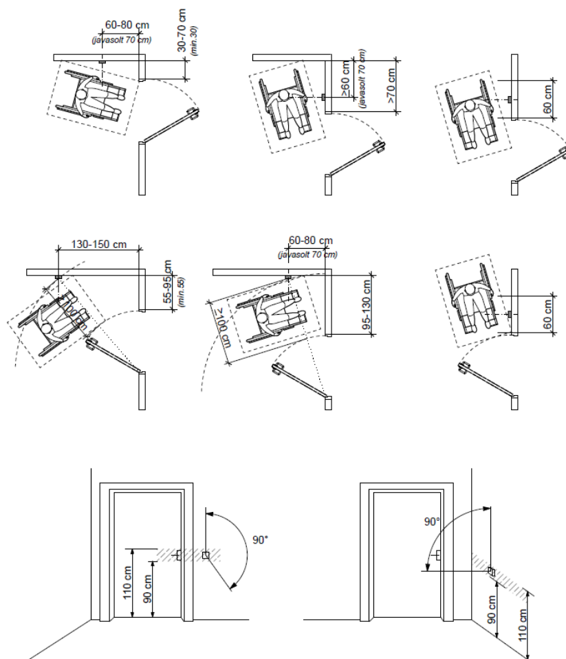
47D ábra: Vésznyitó ajánlott elhelyezési pozíciója
