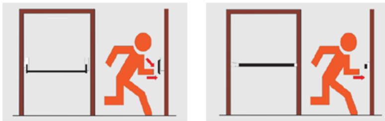
7C ábra: 4 MSZ EN 1125 szerinti pánikajtózár (panic exit device) lenyomós rúddal illetve benyomós rúddal
