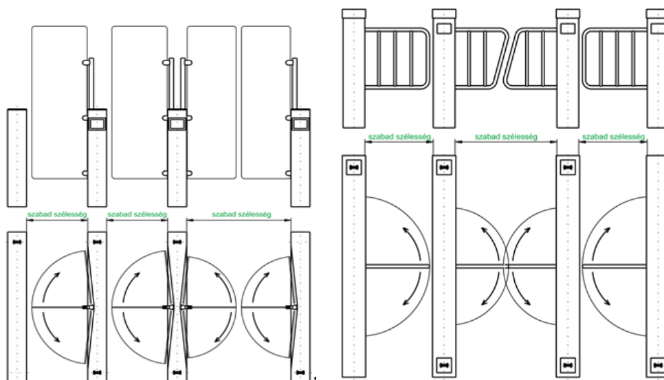
C8. ábra: 3Ajtók szabad szélessége meghatározásának elvei
