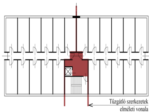
F2.2. ábra Fügőleges tűzszakasz-határral szintenként két tűzszakaszra osztott épület egy átmeneti védett tér és lépcsőház együttesével
