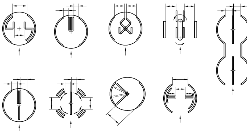
C10. ábra: 4Forgóajtók nyílás szélességének meghatározása
