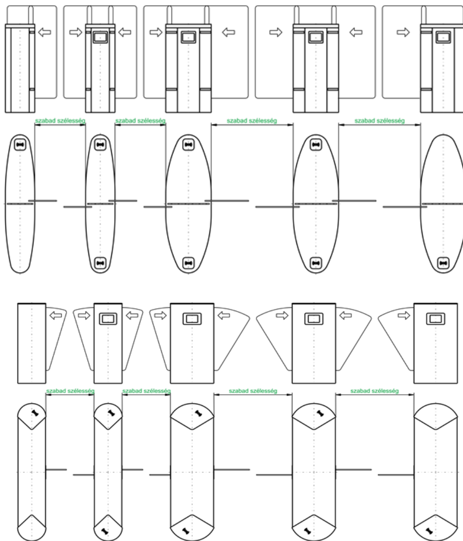
2C9 ábra: Beléptető kapuk szabad nyílásszélességének megállapítása
