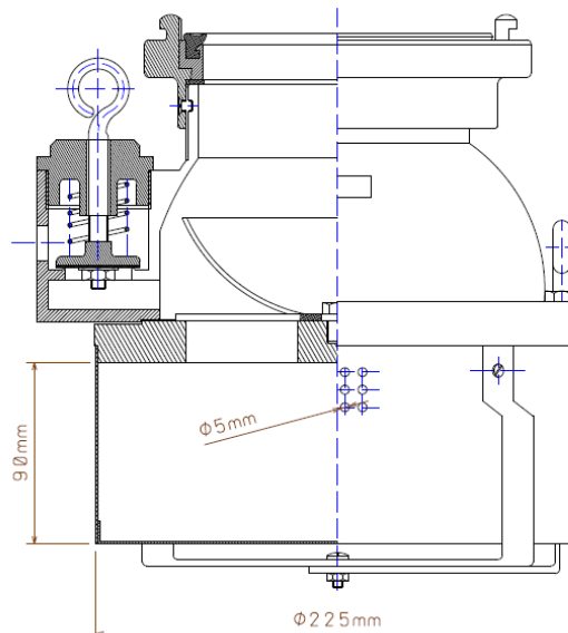
24. 2ábra szűrőkosár
