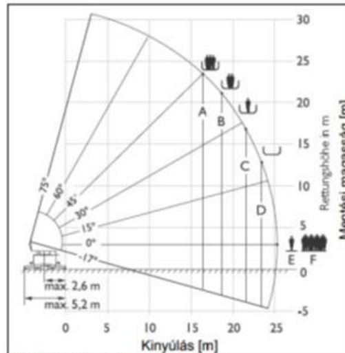
[96] Függőleges használati mező, DLK 23-12 Vario CS 4 tagos létrakészlettel
