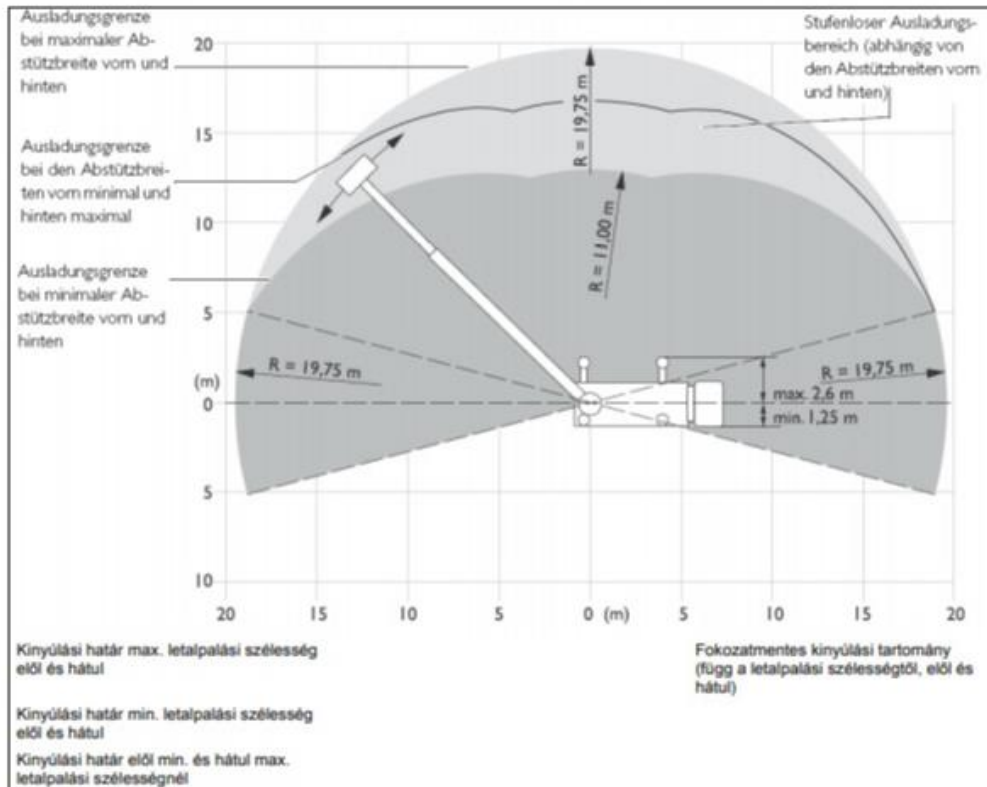
[97] Vízszintes használati mező: kinyúlási határok - példa 3-fős kosárüzemre letalpalási szélességtől
