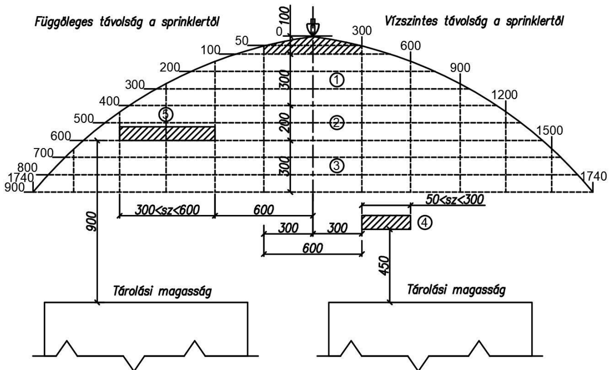
1. ábra ESFR fej szórásképi akadályok
