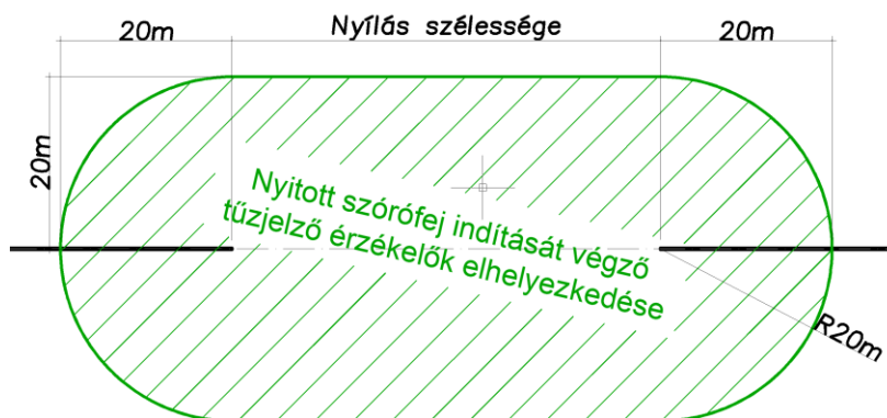
6. ábra: 3 Nytott szórófejes vízfűgöny önműködő indítását végző tűzjelző érzékelők pozíciója
