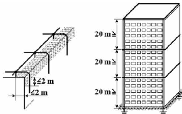
17a. ábra: „L5” fokozatú levezetők kialakítása
