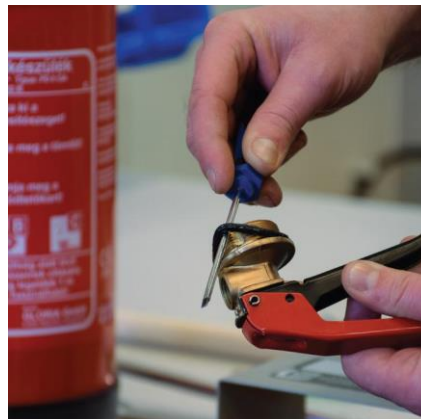
O-gyűrű eltávolítása
